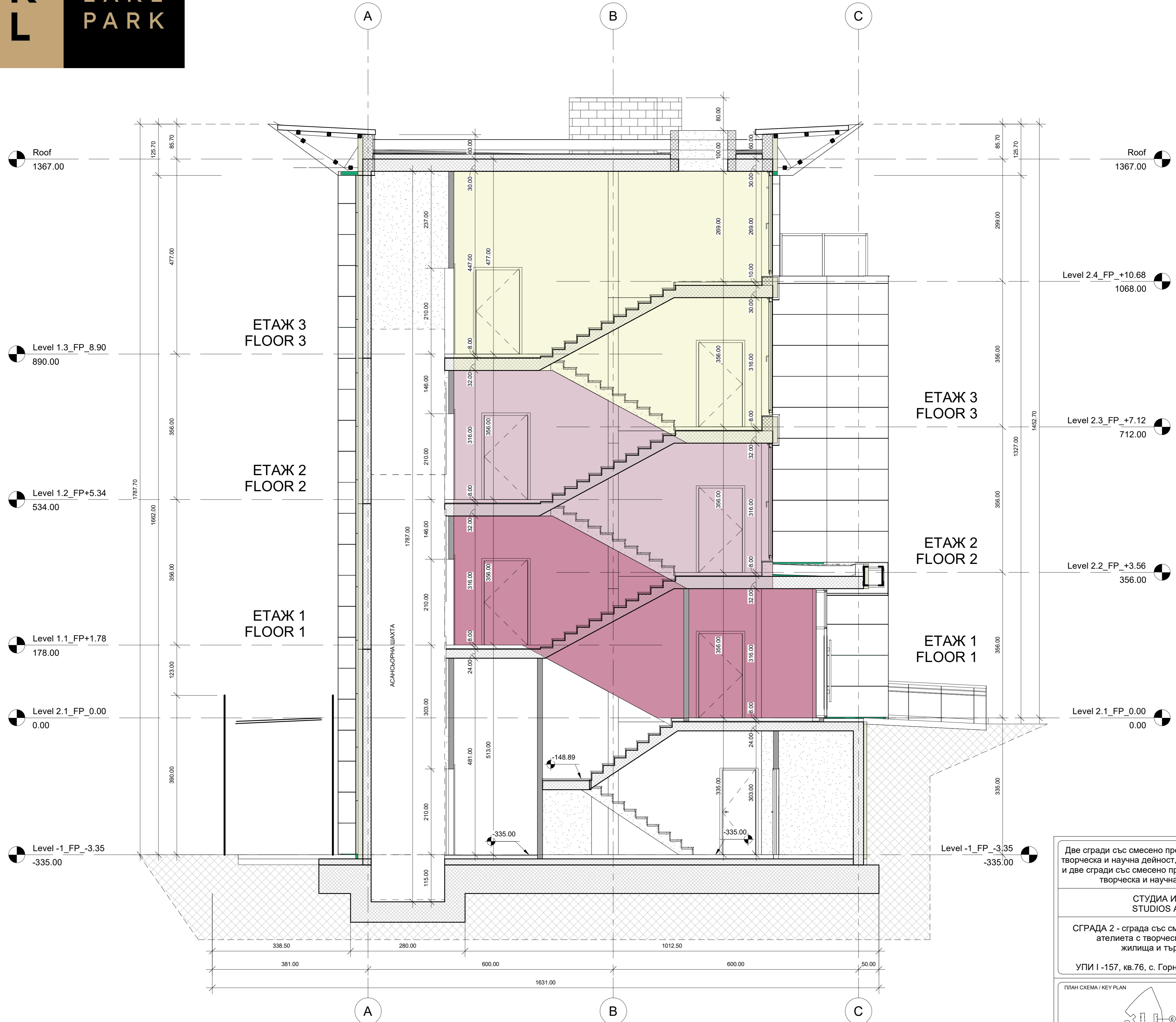
РАЗРЕЗ 1-1 SECTION 1-1
